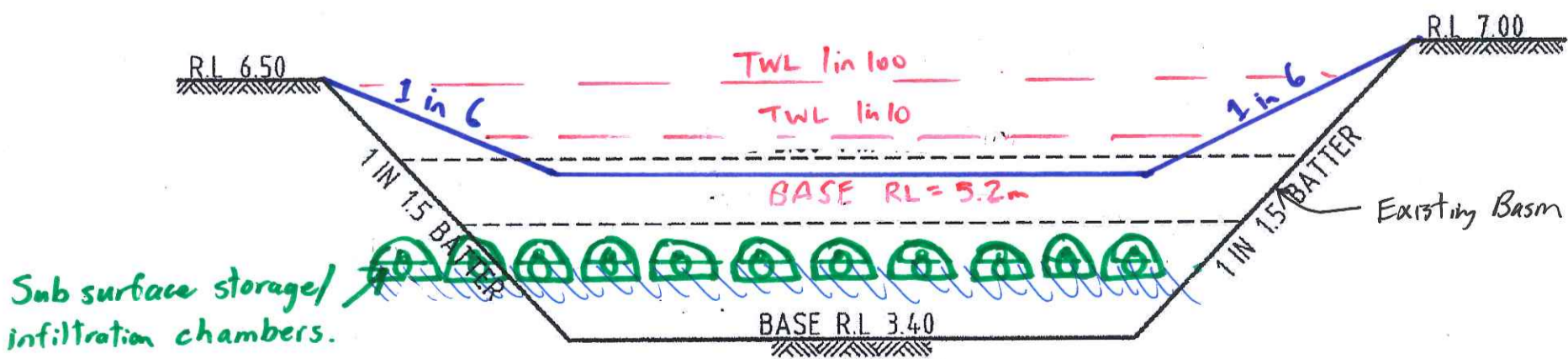
SECTION A-A SCALE 1:200 H 1:100 V
